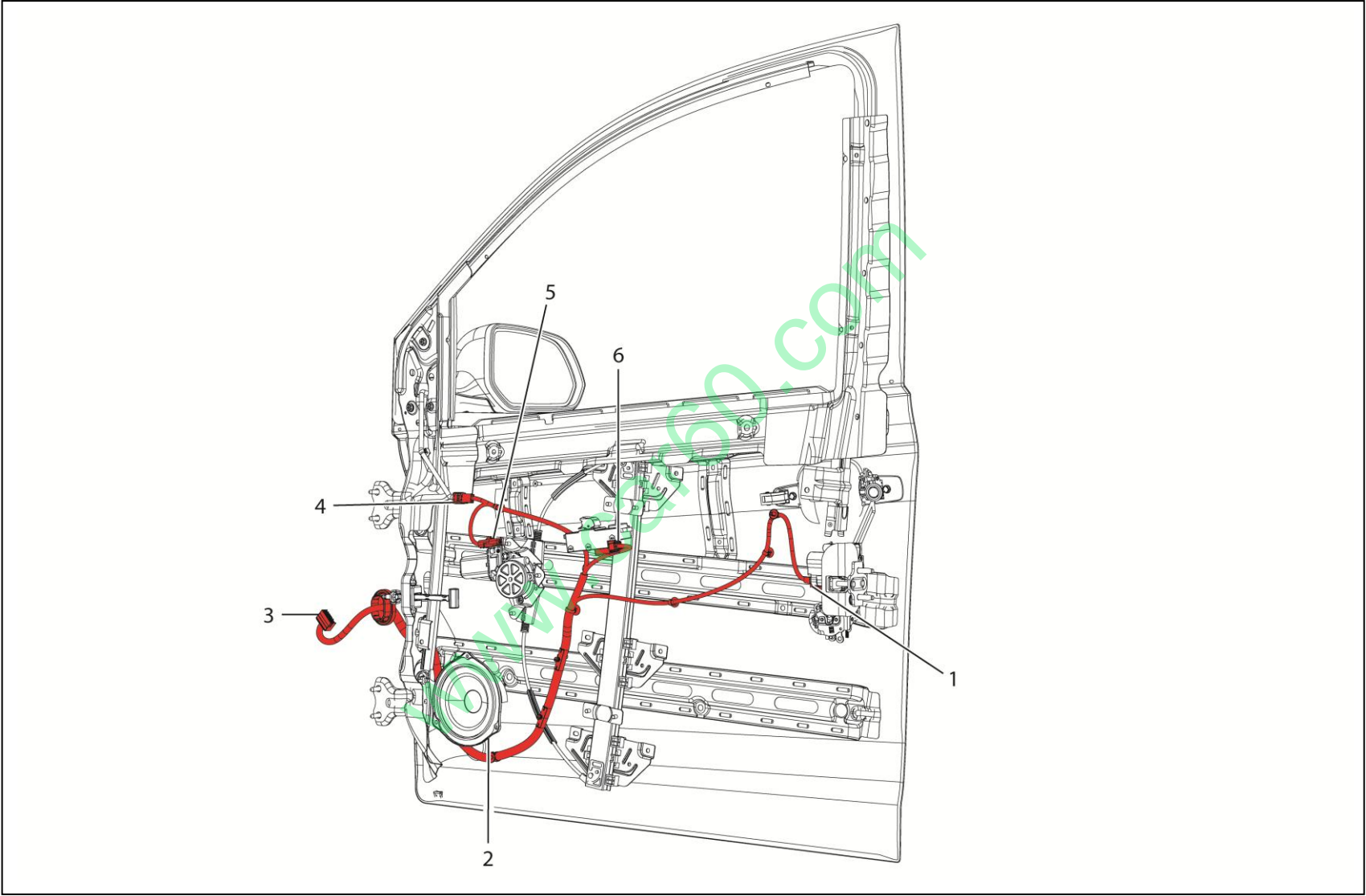
右前门线束
